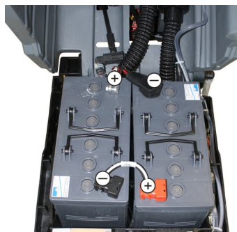
Esquema de montaje para 2 baterías
