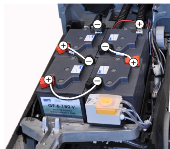
Esquema de montaje para 4 baterías
